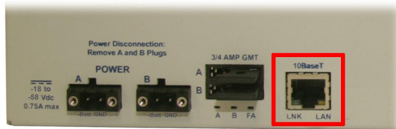
Fig. 5.3 LAN Port
